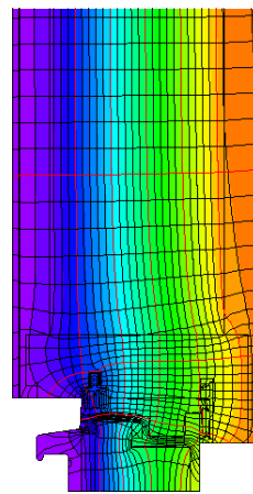
Isothermengrafik
